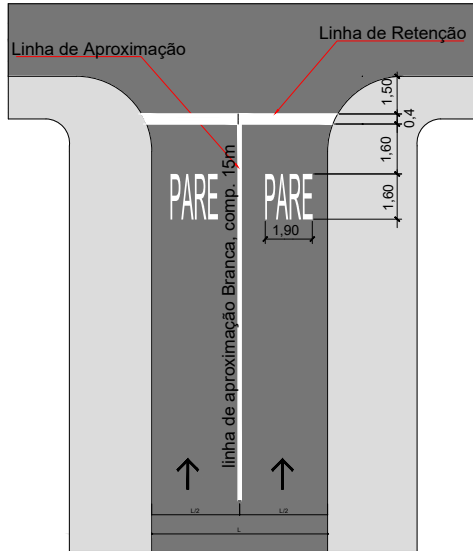
Legenda PARE, Linha de Retenção e Linha de Aproximação
