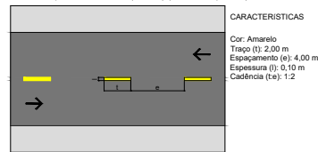
Linha Simples Seccionada (LFO-2) (sentidos opostos)
