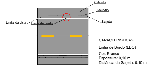
Linha de Bordo (LBO) Duas faixas em cada rua indicada
